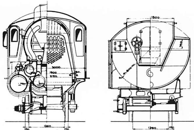
Ritning i skala 1:87 av lokomotiv och tender litt. F kompletterad med några närbilder av nr 1200.
