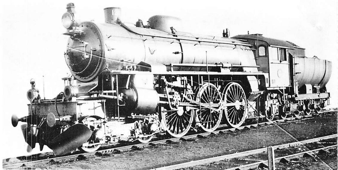
Axelboxarna på boggien och på tendern levererades med SKF kullager, vilket föranledde SKF att ta denna sällan publicerade bild av F nr 1200. Kullagren, tydligen före sin tid, utbyttes senare mot glidlager.
