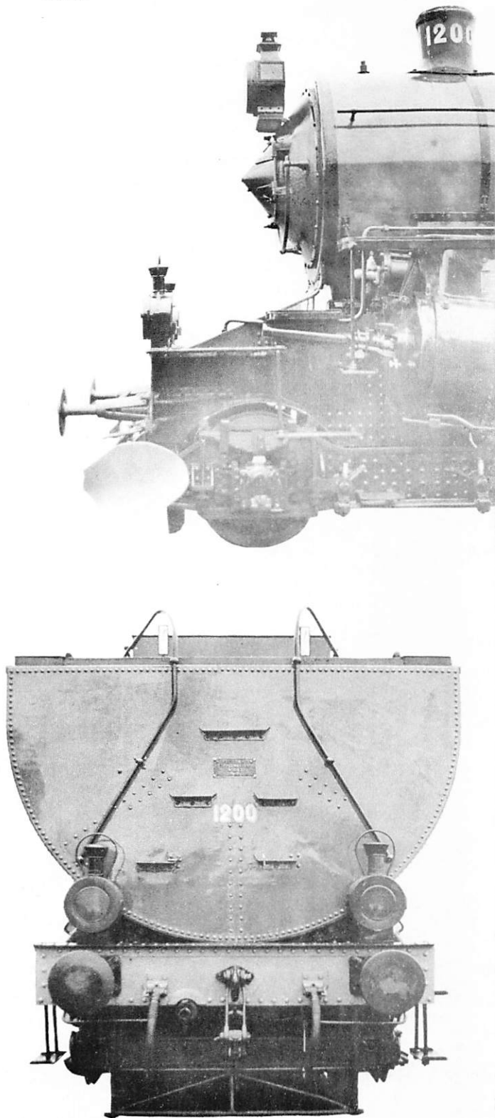
Ritning i skala 1:87 av lokomotiv och tender litt. F kompletterad med några närbilder av nr 1200.
